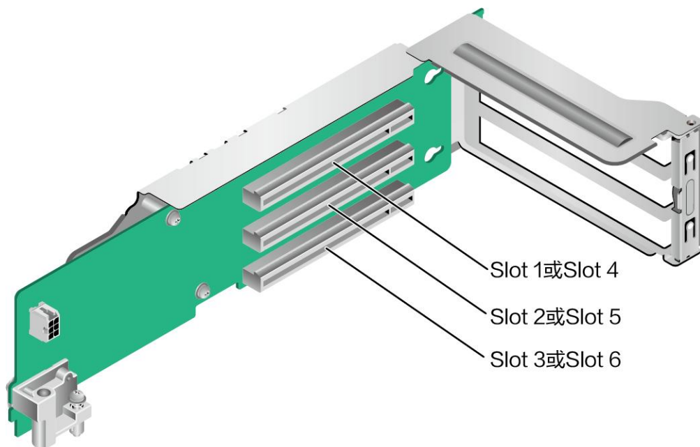
图 5-21 3*x8 Riser 卡
