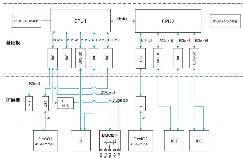
图 4-1 逻辑结构
