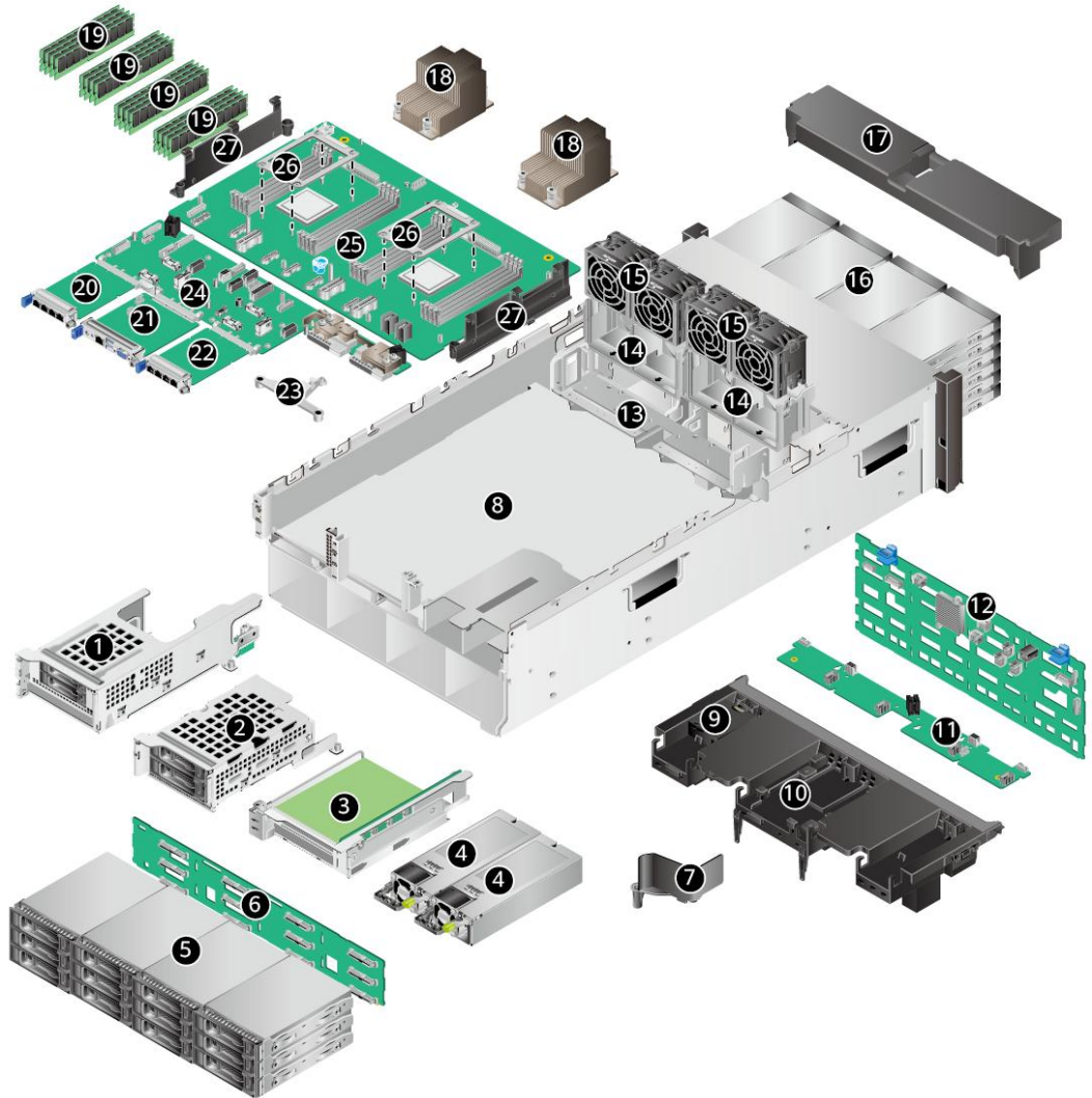
图 3-1 部件
