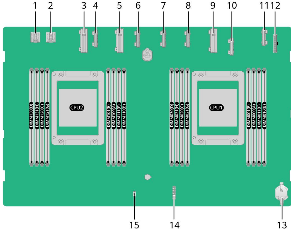
图 5-3 基础板接口
