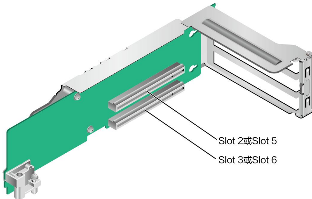
图 5-22 2*x8 Riser 卡
