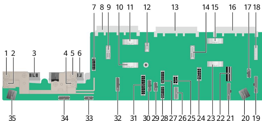
图 5-5 扩展板
