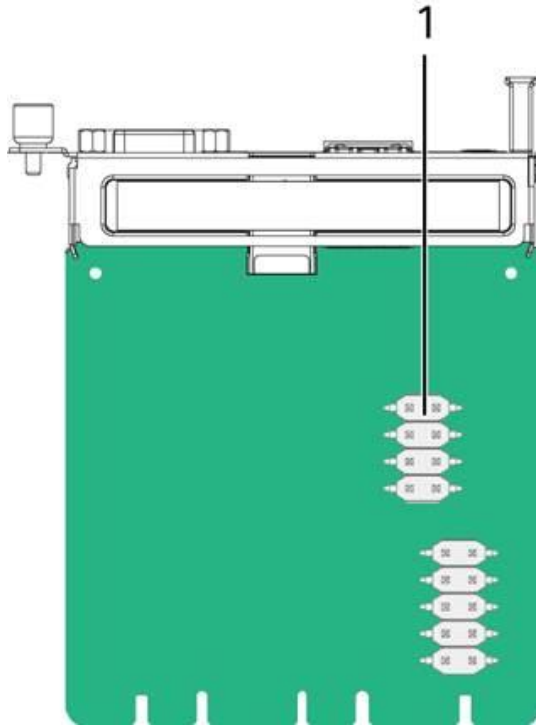
图 5-29 BMC 插卡
