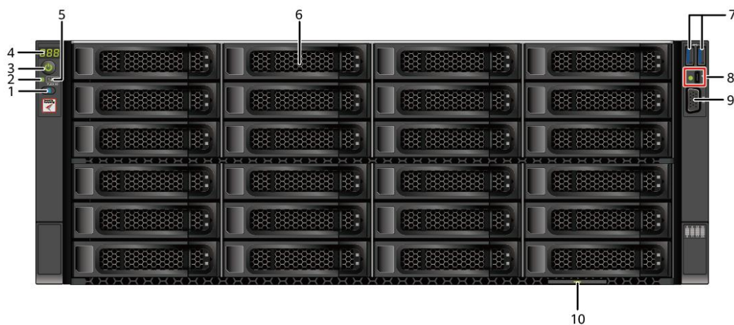
图 6-1 36x3.5 英寸硬盘配置前面板
