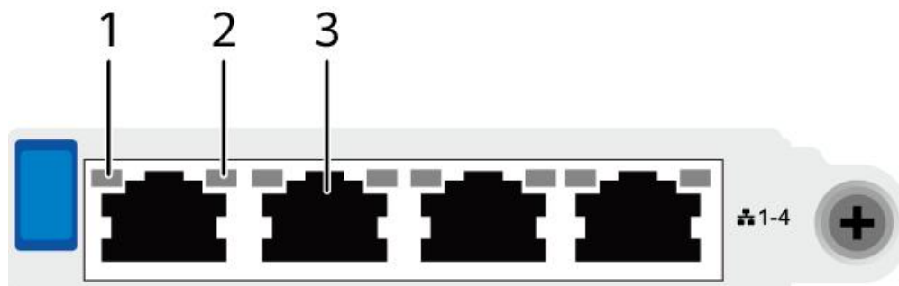
图 6-25 SF221Q (4xGE 电口)
