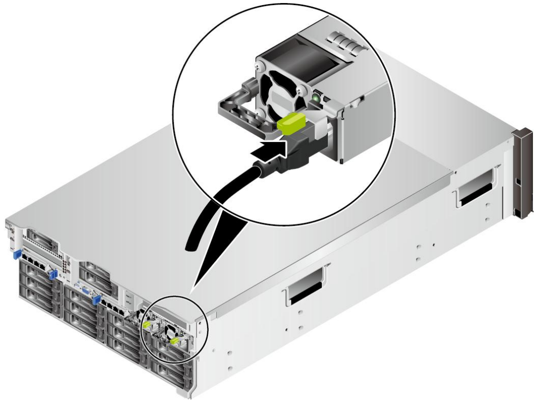
图 9-26 连接电源线缆
