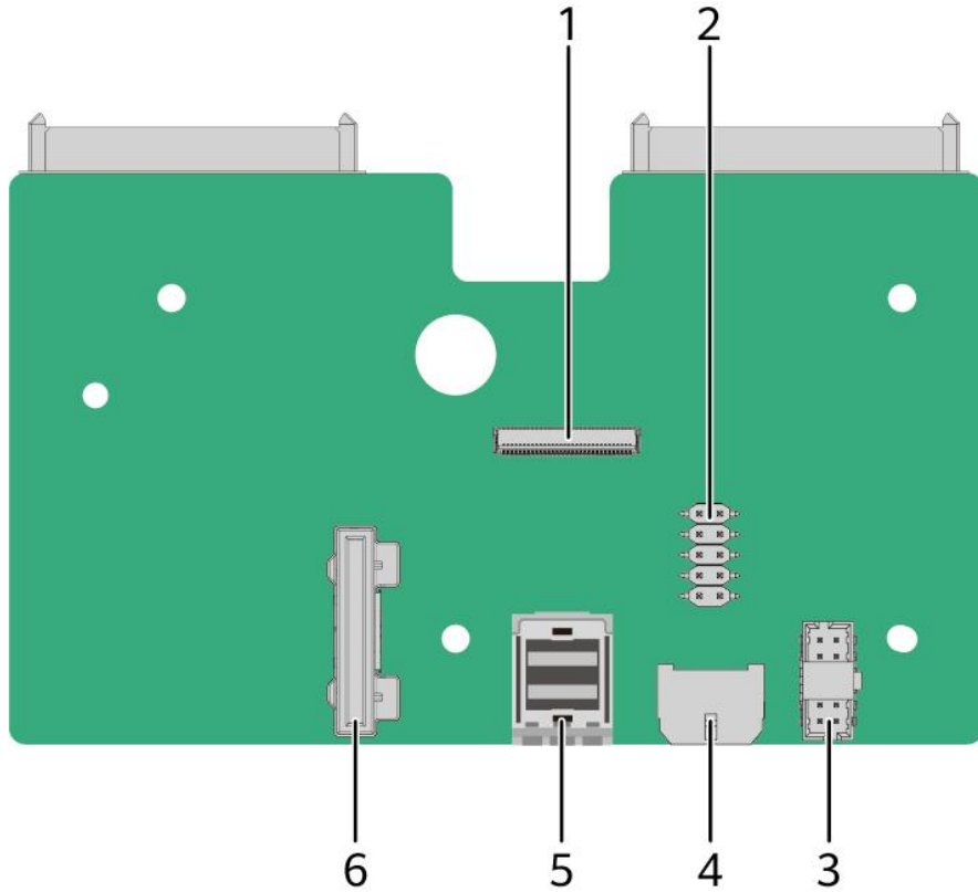
图 6-19 IO 模组 3 水平硬盘背板（下板）
