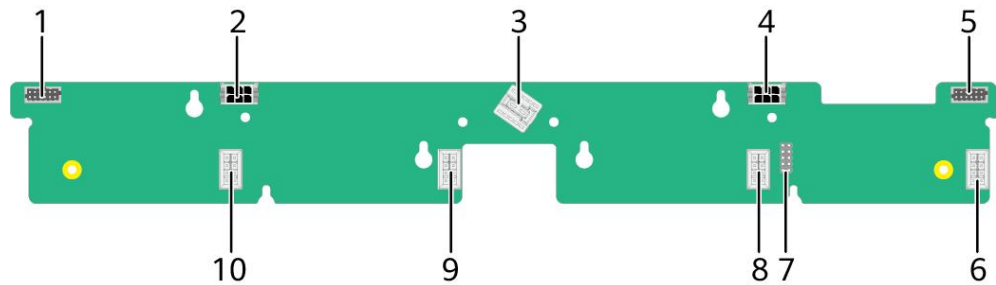
图 6-6 风扇板接口
