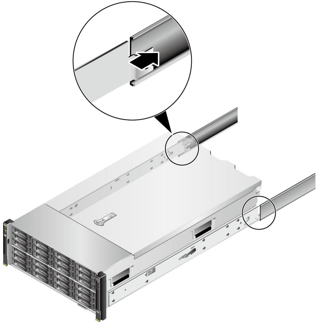
图 9-14 安装服务器
