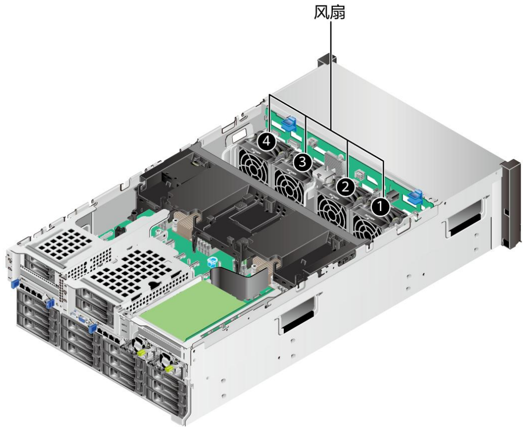
图 6-7 风扇位置图
