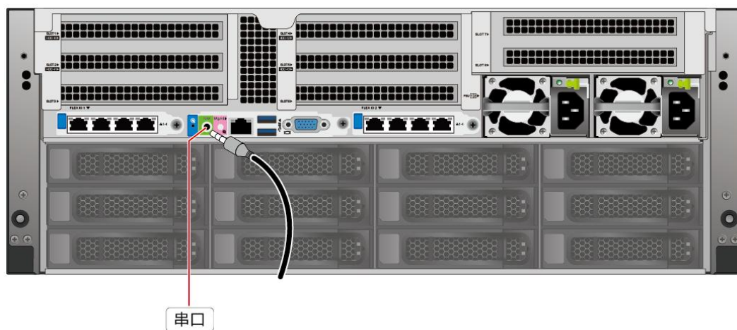
图 9-25 连接串口线缆
