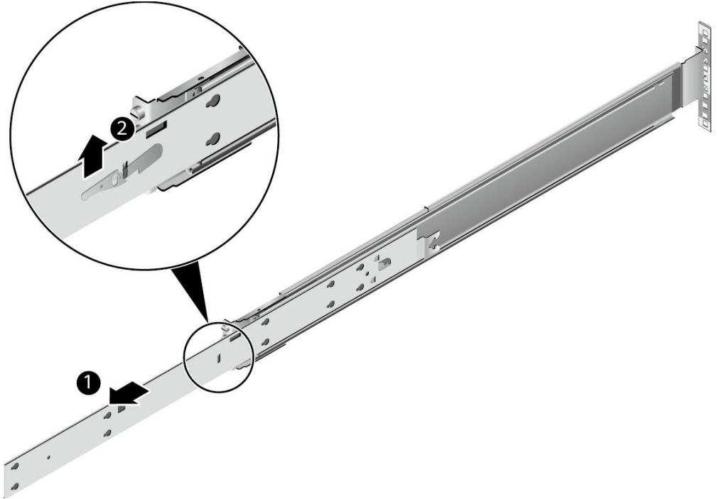
图 9-12 抽出内轨
