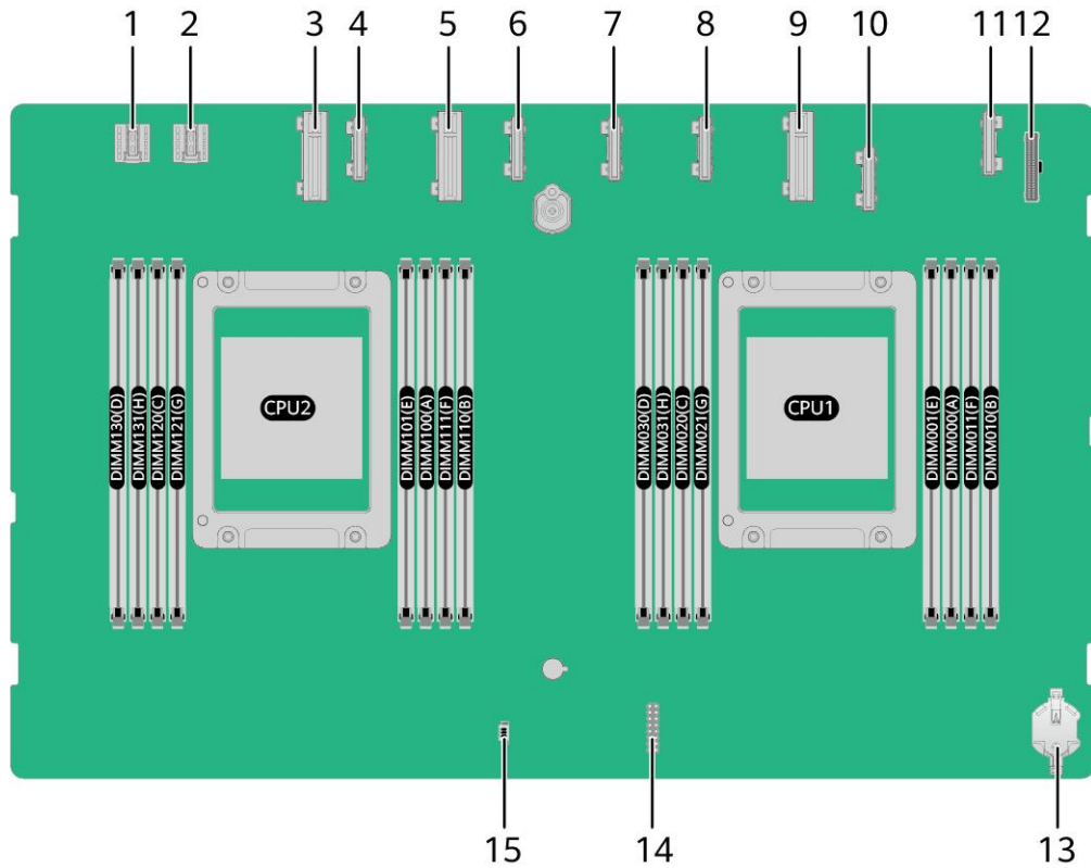
图 6-3 基础板接口
