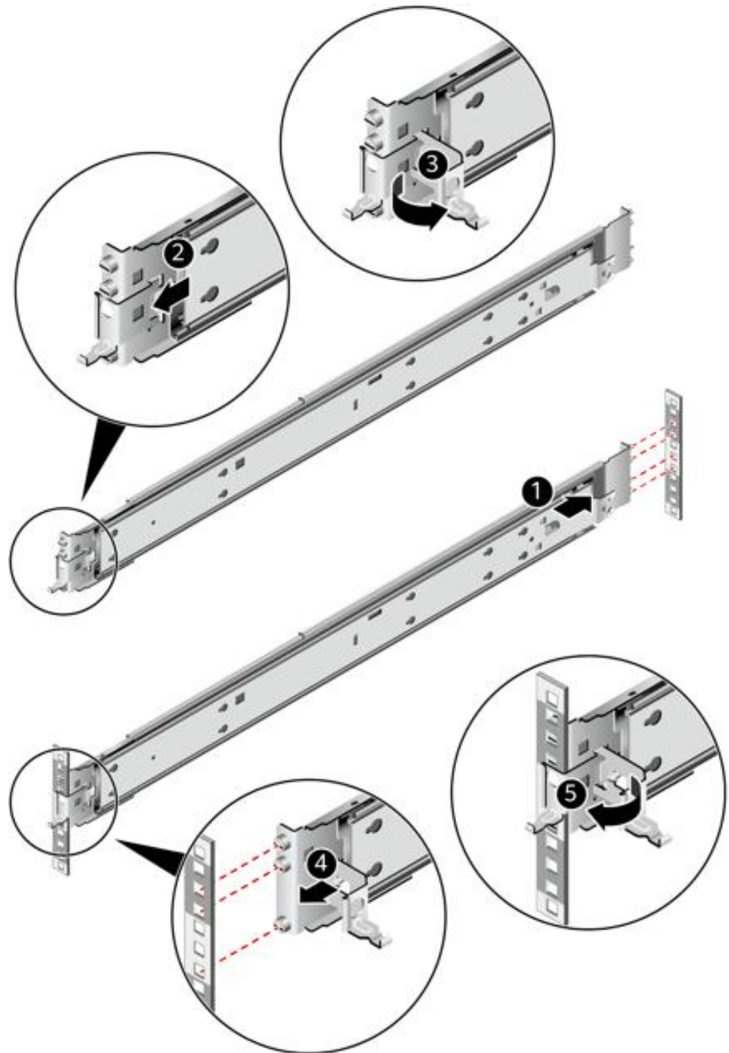
图 9-11 安装抱轨
