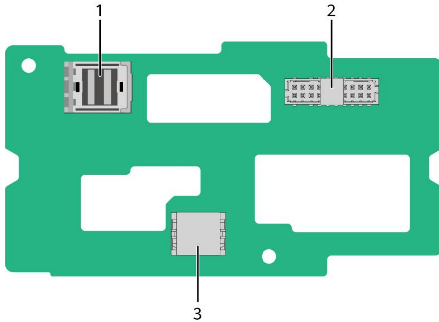
图 6-16 2x3.5 英寸后置硬盘背板
