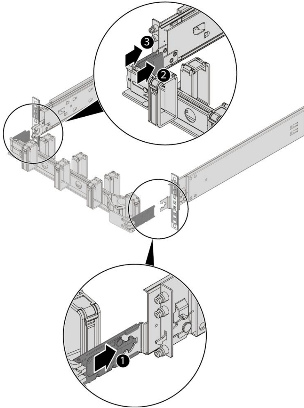
图 9-17 安装理线架
