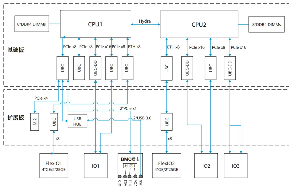
图 5-1 逻辑结构
