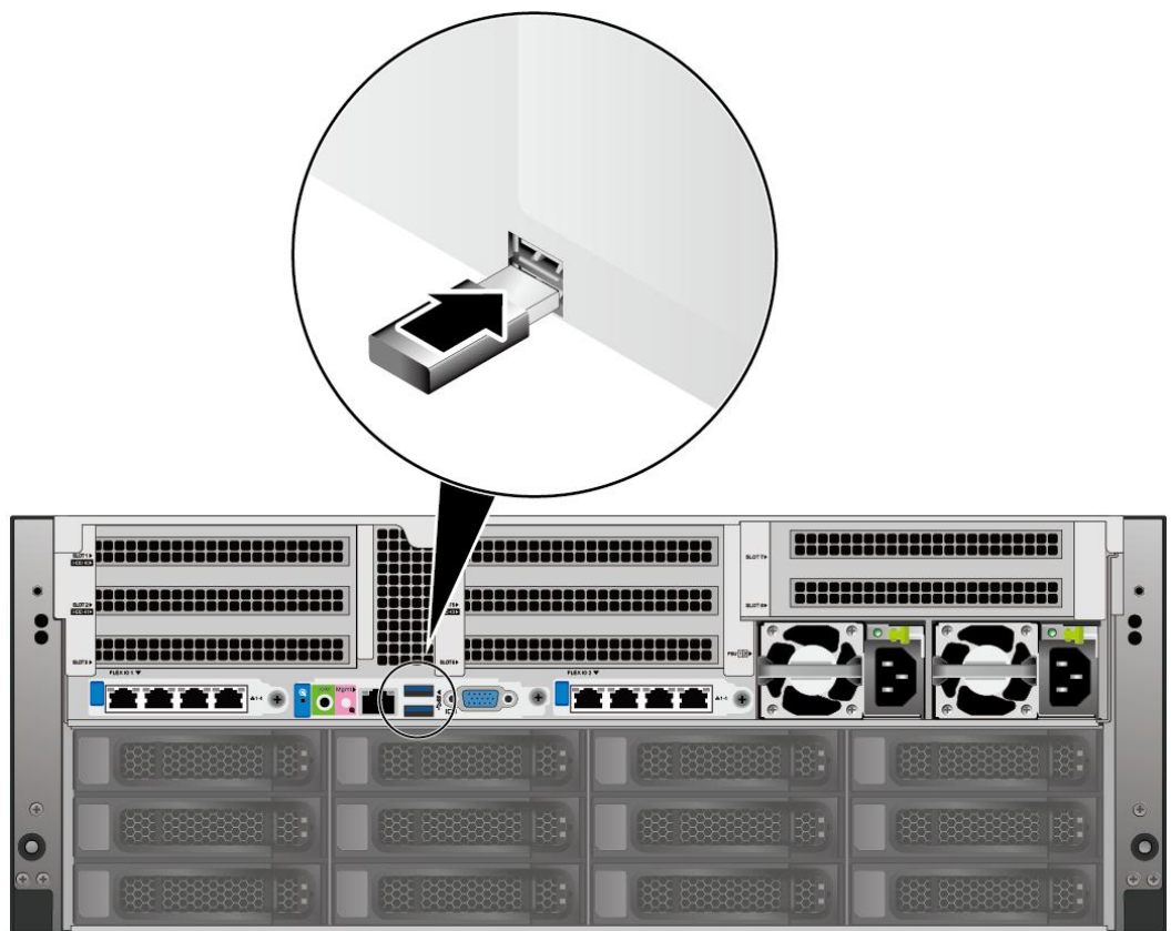
图 9-24 连接 USB 接口
