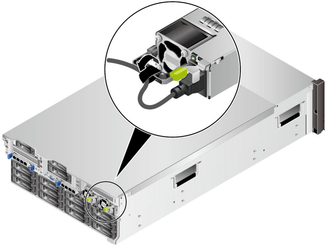
图 9-27 固定电源线缆
