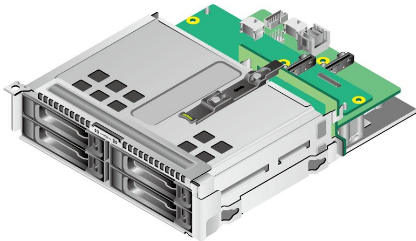
图 6-13 后置 4x2.5 英寸硬盘模组
