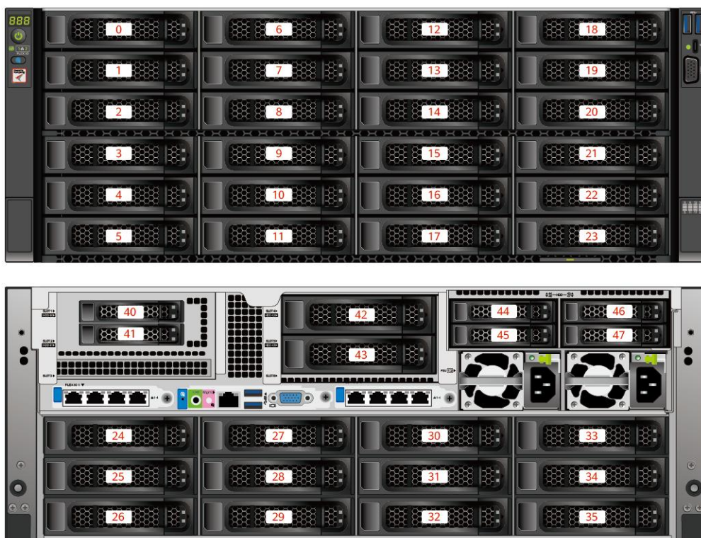
图 6-8 36x3.5 英寸硬盘 EXP 配置硬盘编号
