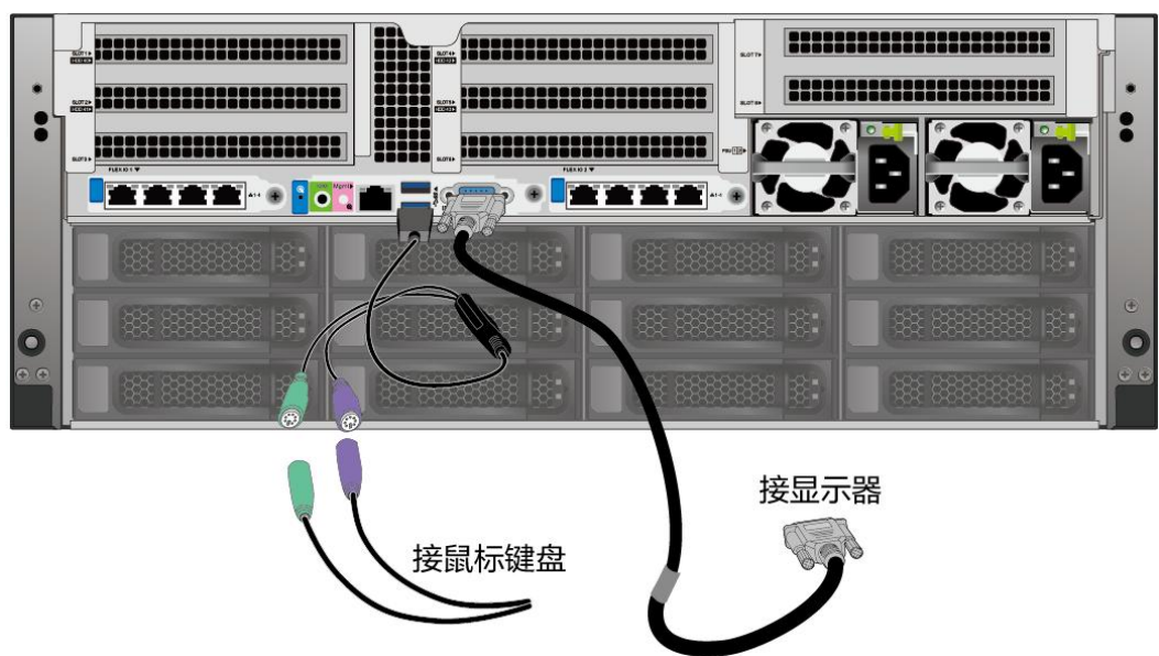
图 9-18 连接 USB 转 PS2 线缆和 VGA 接口
