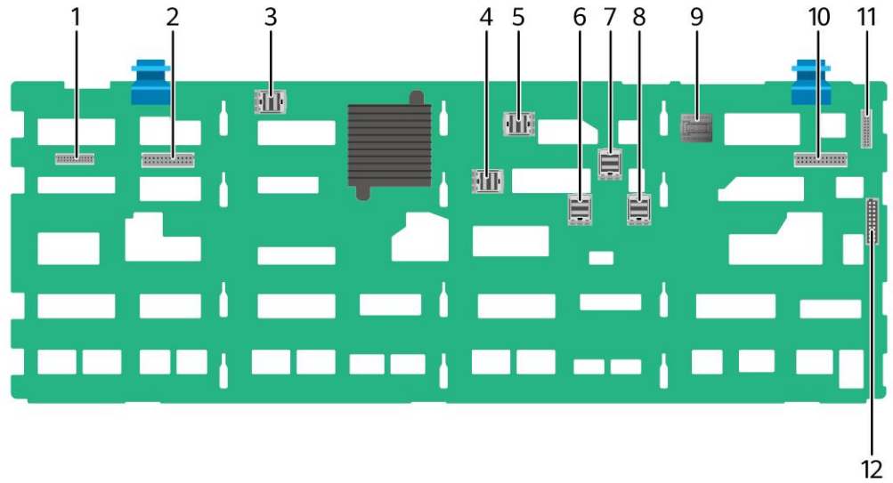
图 6-14 24x3.5 英寸硬盘 EXP 配置硬盘背板
