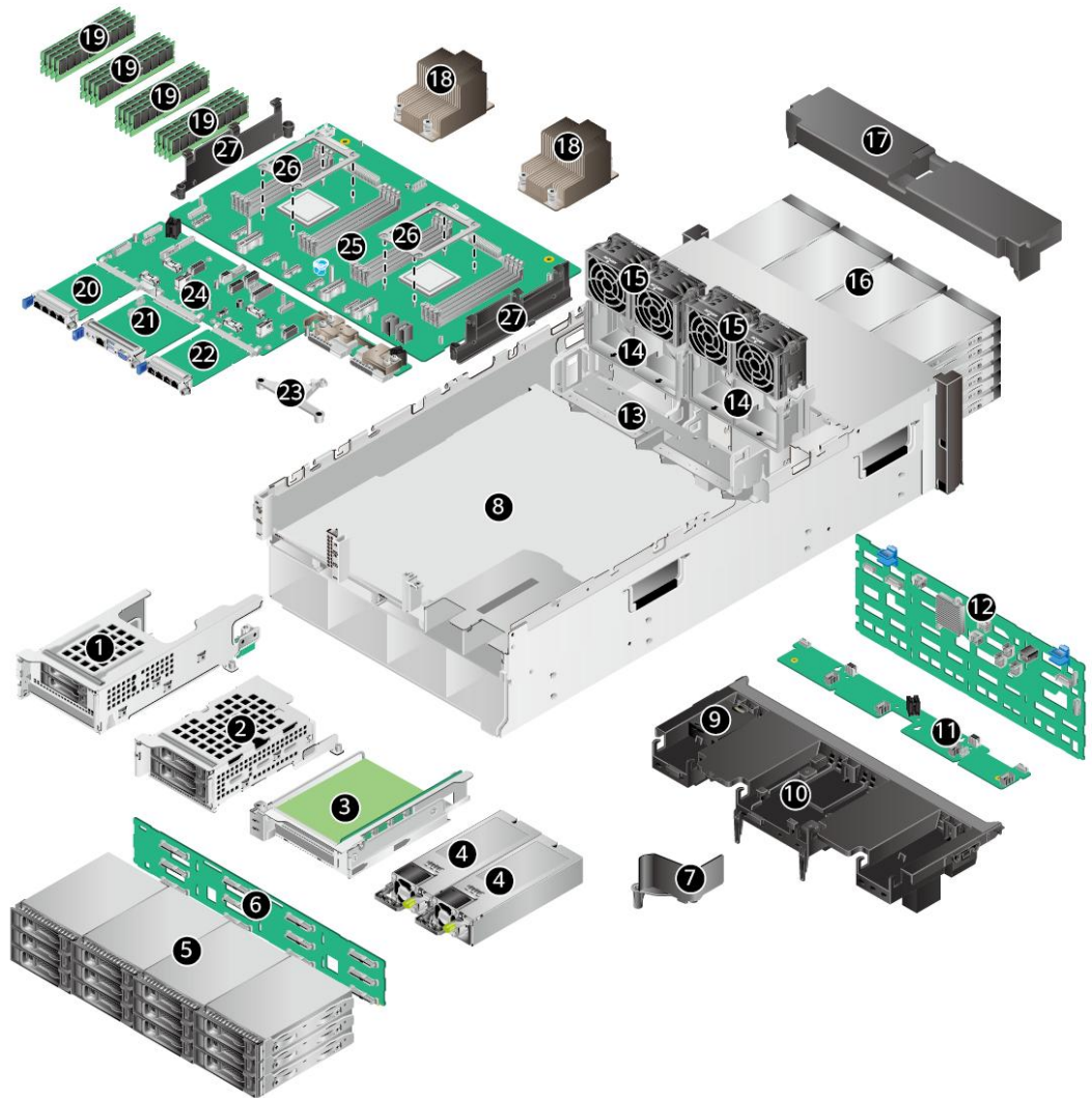
图 4-1 部件
