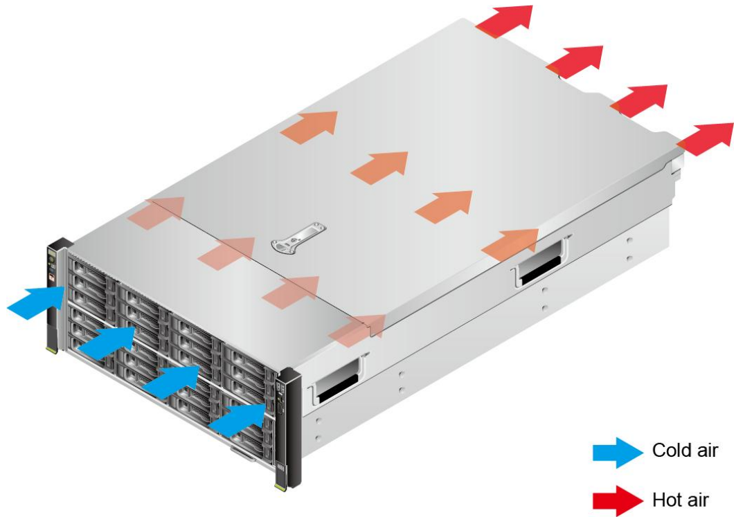
图 9-4 散热气流走向示意图
