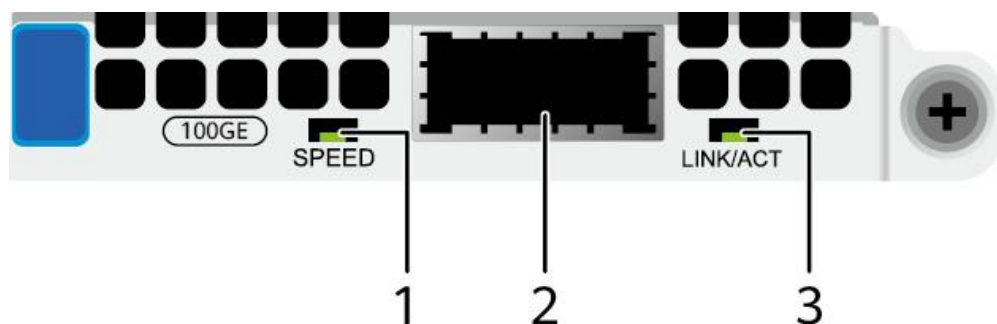
图 6-27 SF225S-H (1x100GE 光口)
