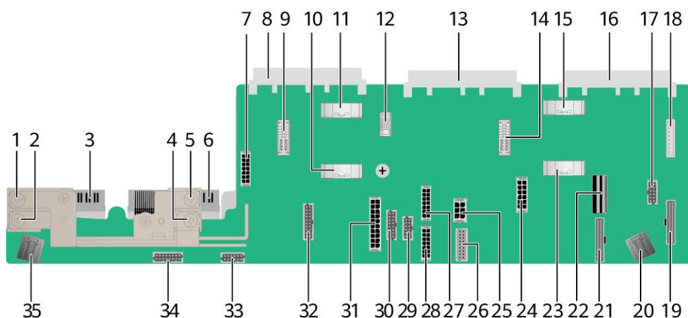
图 6-5 扩展板
