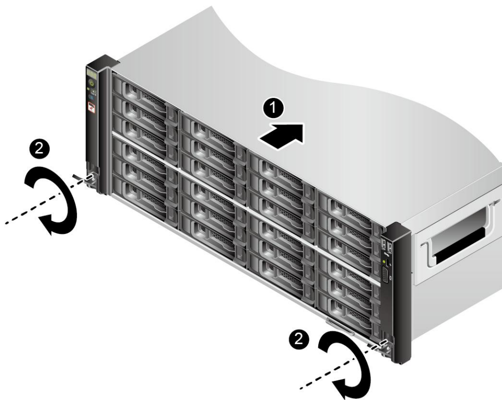
图 9-10 安装服务器
