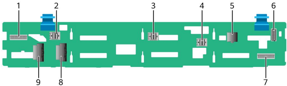
图 6-15 12x3.5 英寸后置硬盘背板
