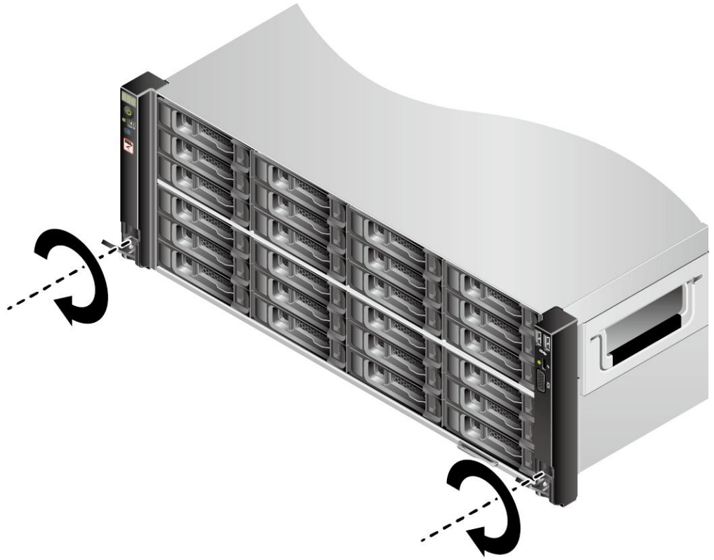
图 9-16 固定服务器
