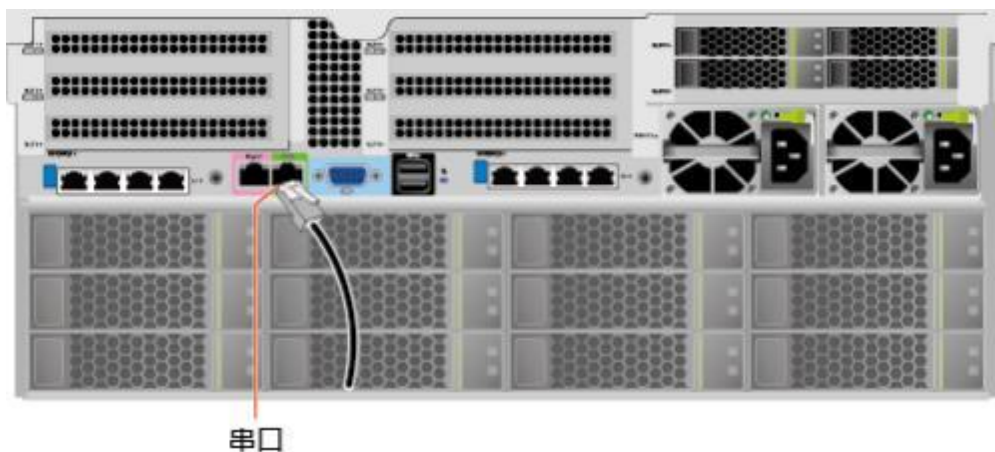
图 6-18 连接串口线缆
