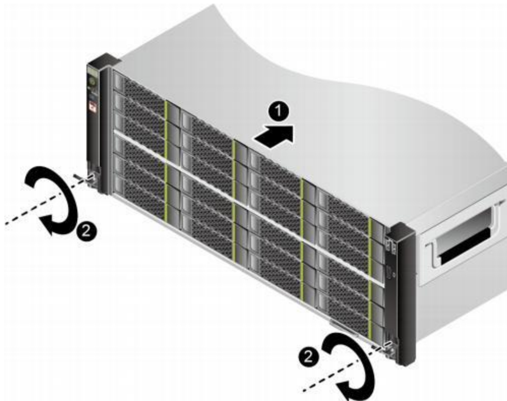
图 6-7 安装服务器
