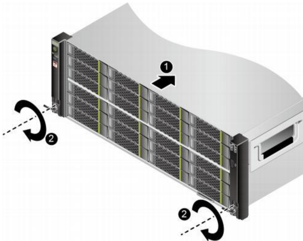
图 6-11 安装服务器
