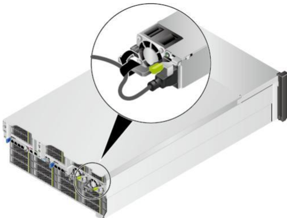
图 6-20 固定电源线缆
