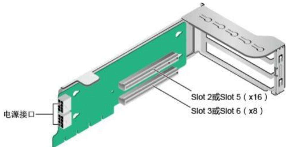
图 3-11 Riser 卡 2 ( 1x8+1x16)
