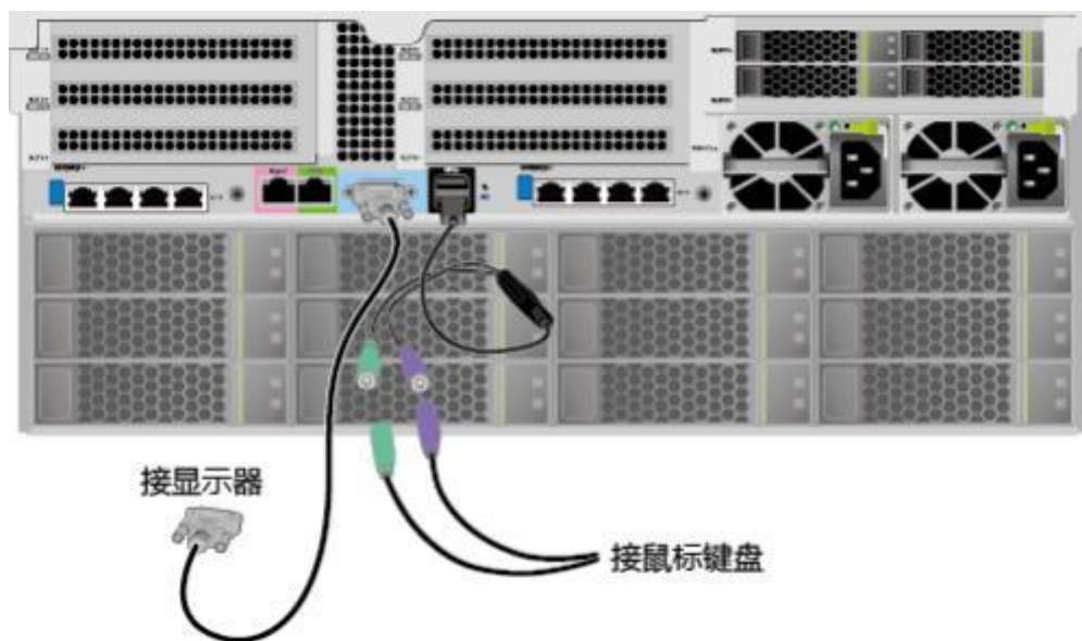
图 6-12 连接 USB 转 PS2 线缆和 VGA 接口
