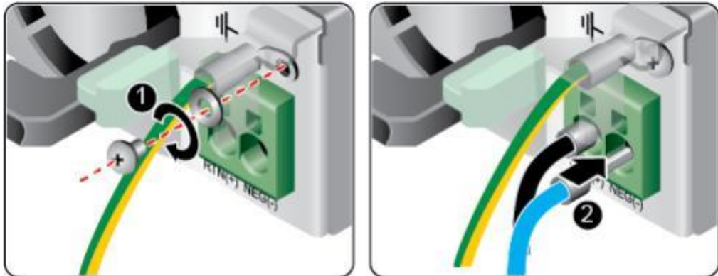
图 6-21 连接线缆
