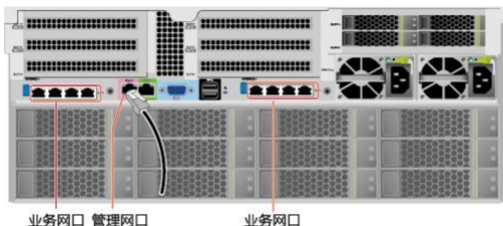
图 6-13 连接网线
