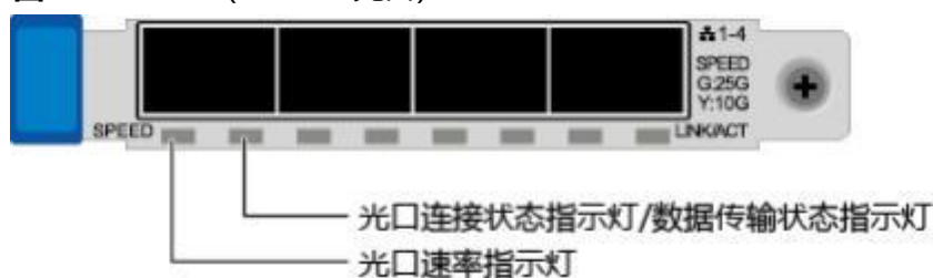
图 3-6 TM280 (4x25GE 光口)
