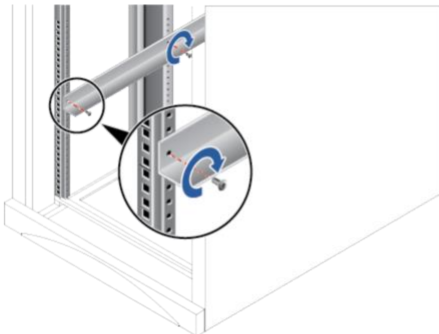
图 6-6 安装 L 型滑道
