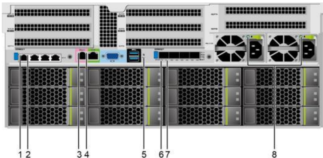
图 3-4 后面板指示灯
