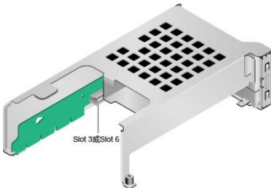
图 3-12 Riser 卡 3 ( 1x16)
