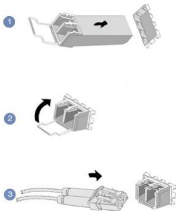
图 6-14 连接光纤
