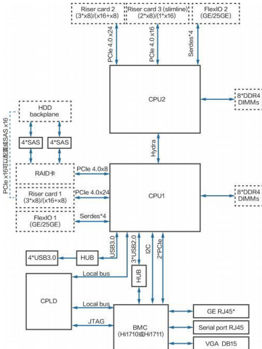
图 2-3.2 服务器逻辑结构
