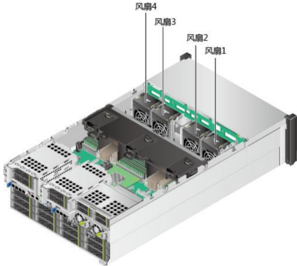
图 3-17 风扇位置图
