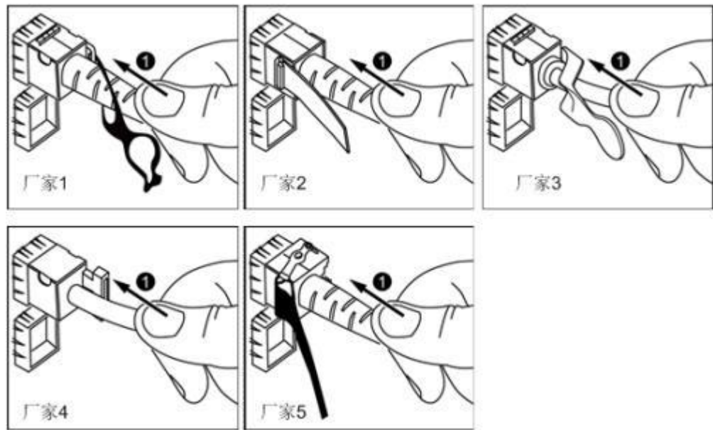
图 6-16 连接 SFP+电缆
