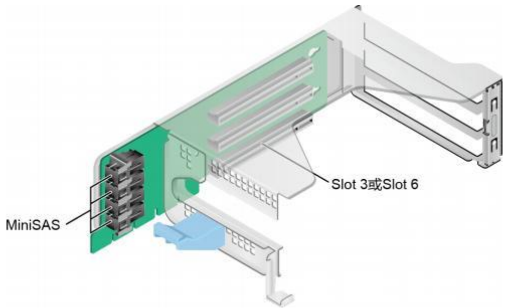
图 3-13 Riser 卡 4 ( SAS Riser)
