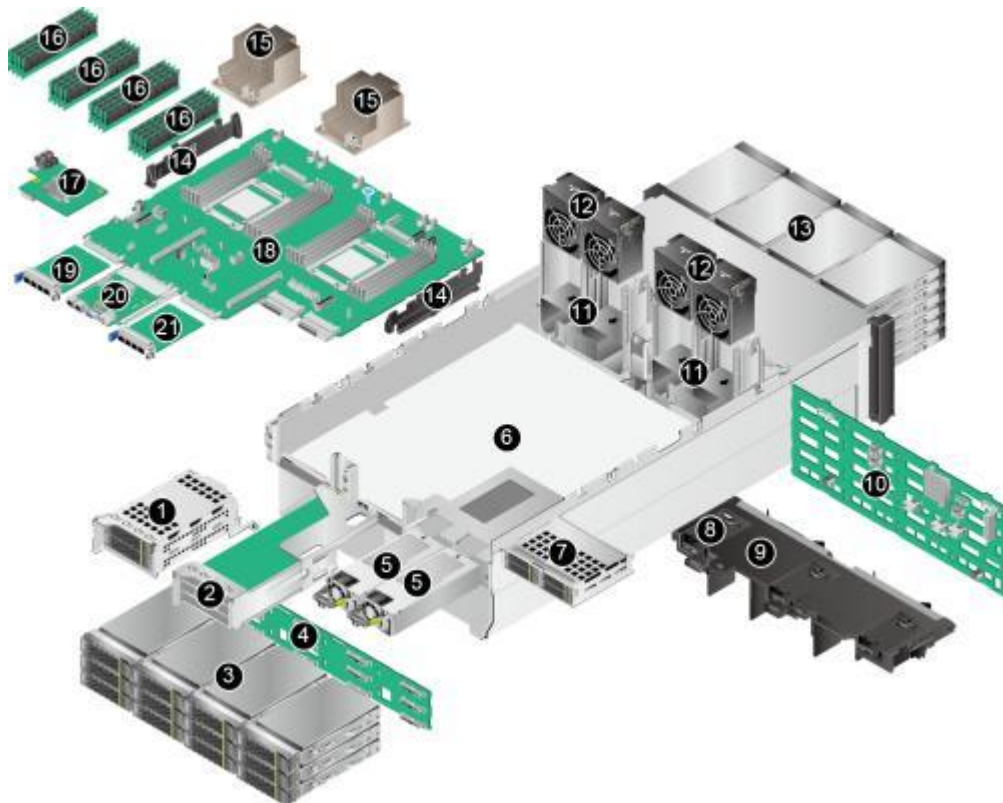
图 2-2.2 部件(配置鲲鹏920 5220、5221K、3210、3211K 处理器)
