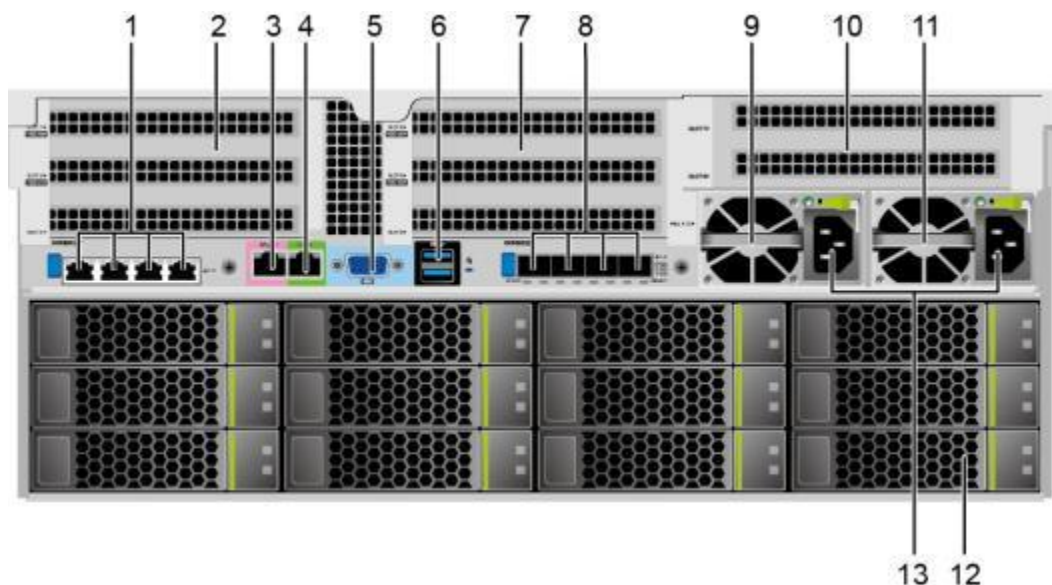
图 3-3 后面板组件
