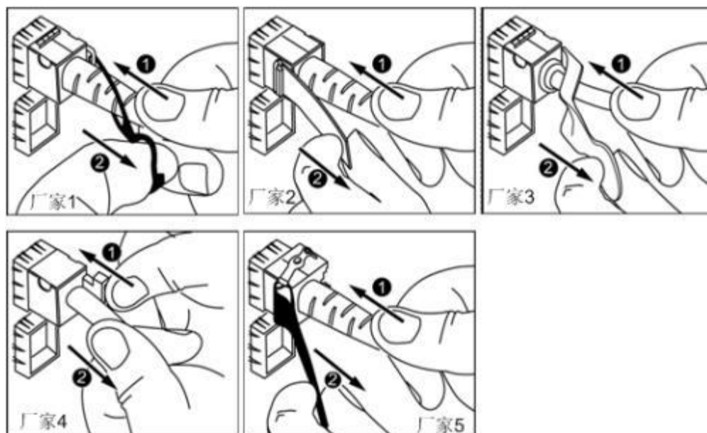
图 6-15 拔出 SFP+ 电缆
