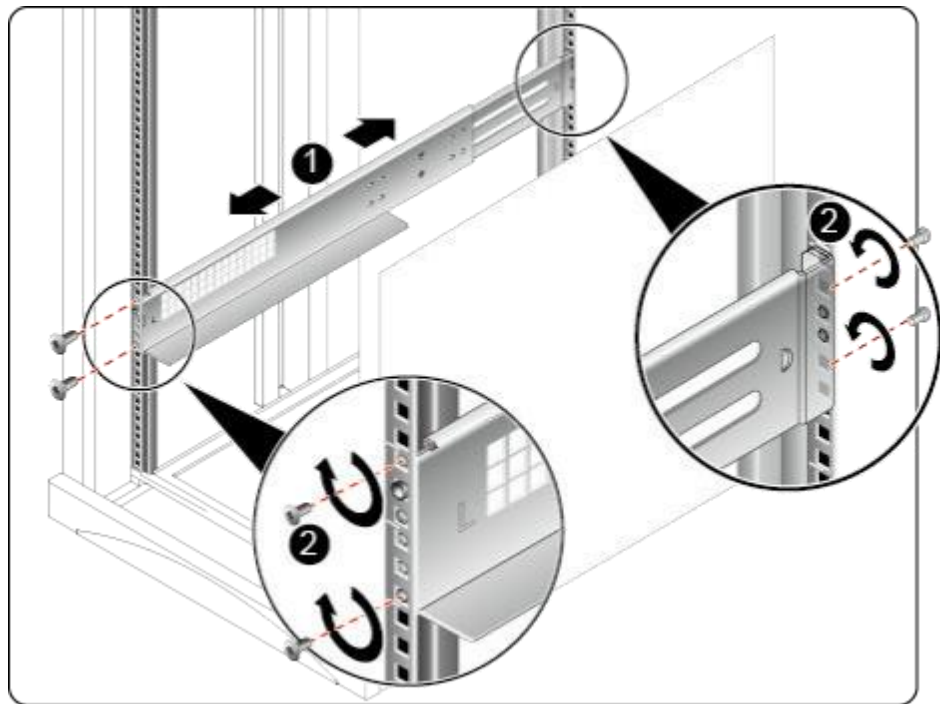
图 6-10 安装可伸缩滑道
