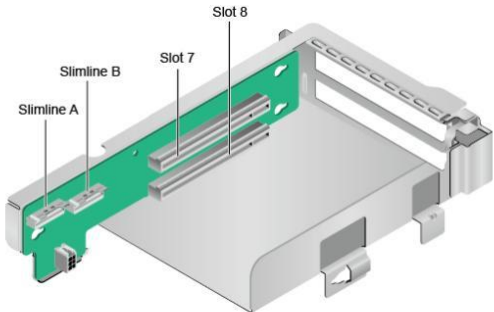
图 3-14 Riser 卡 5 (2x8)
