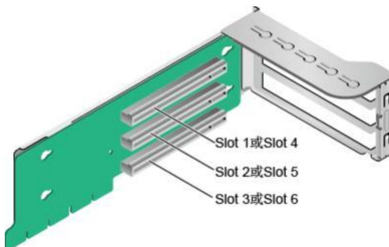
图 3-10 Riser 卡 1 (3x8)
