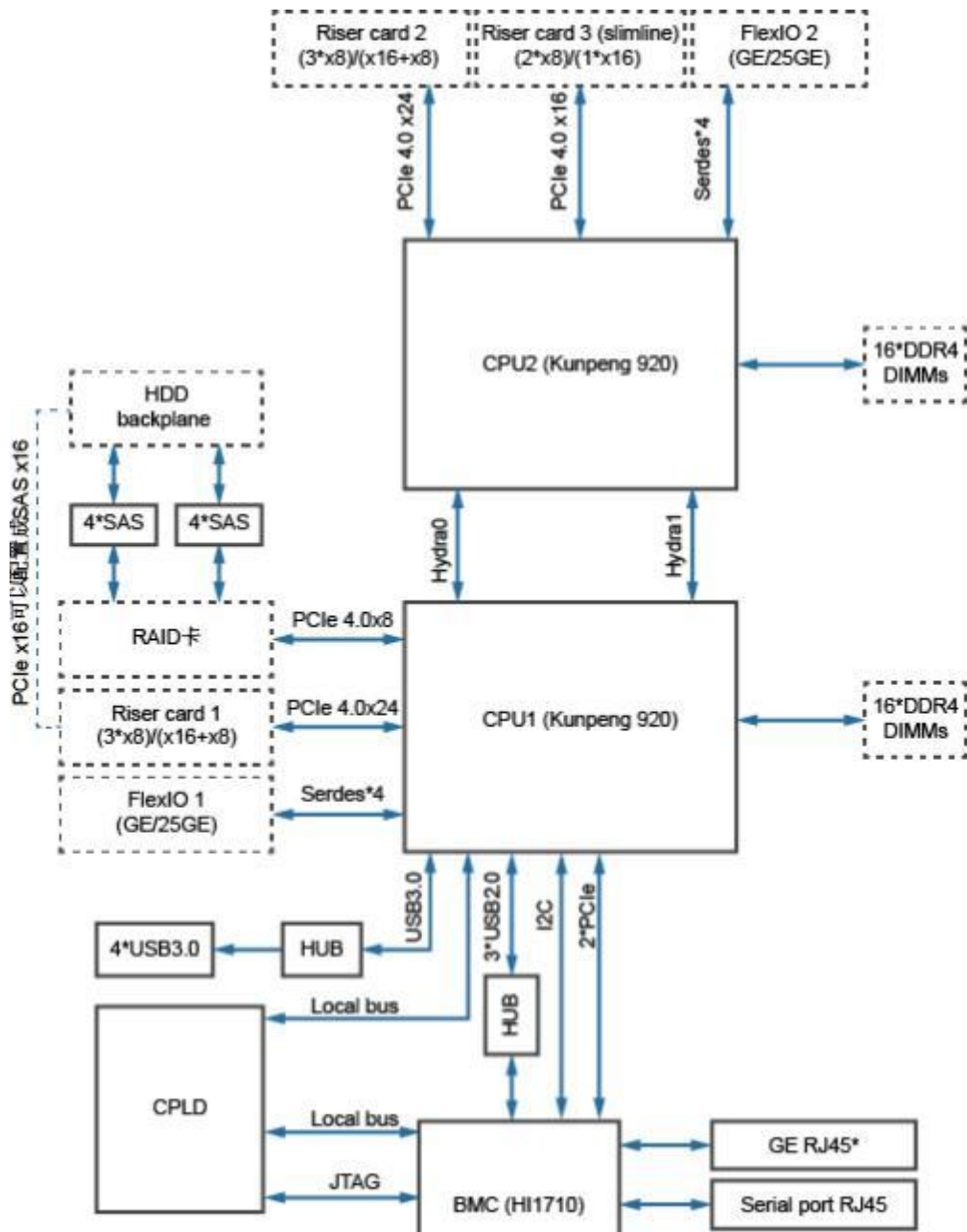
图 2-3.1 服务器逻辑结构
