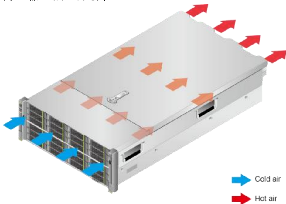
图 6-3 散热气流走向示意图
