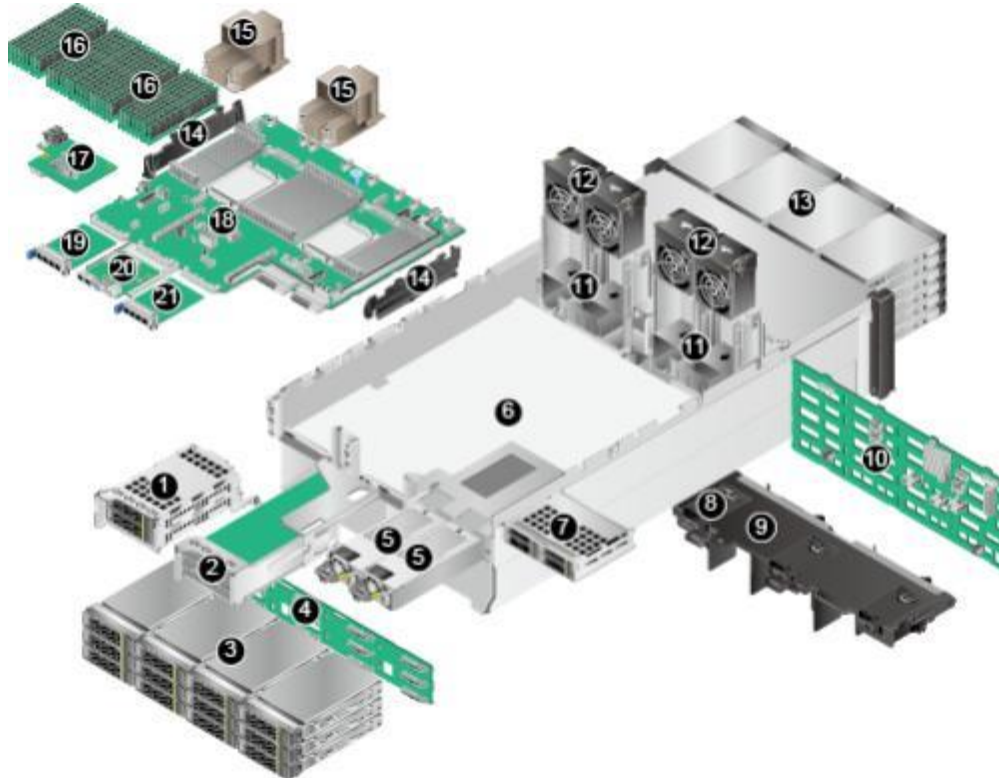
图 2-2.1 部件(配置鲲鹏 920 920 7260、7261K、5250、5251K 处理器)
