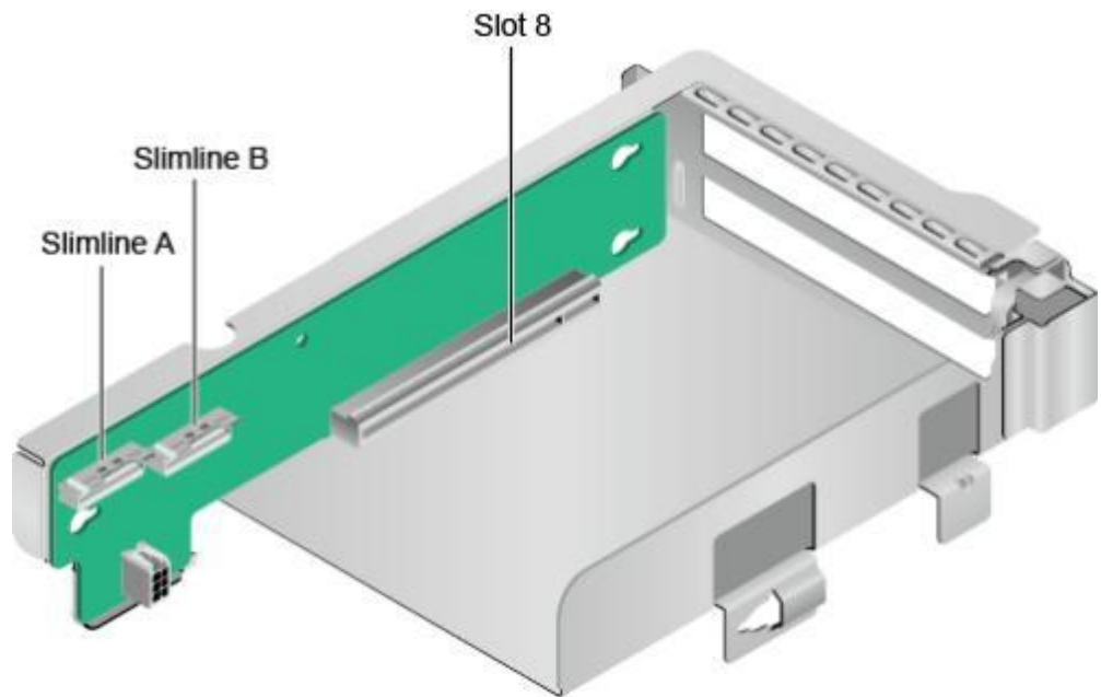
图 3-15 Riser 卡 6 (1x16)
